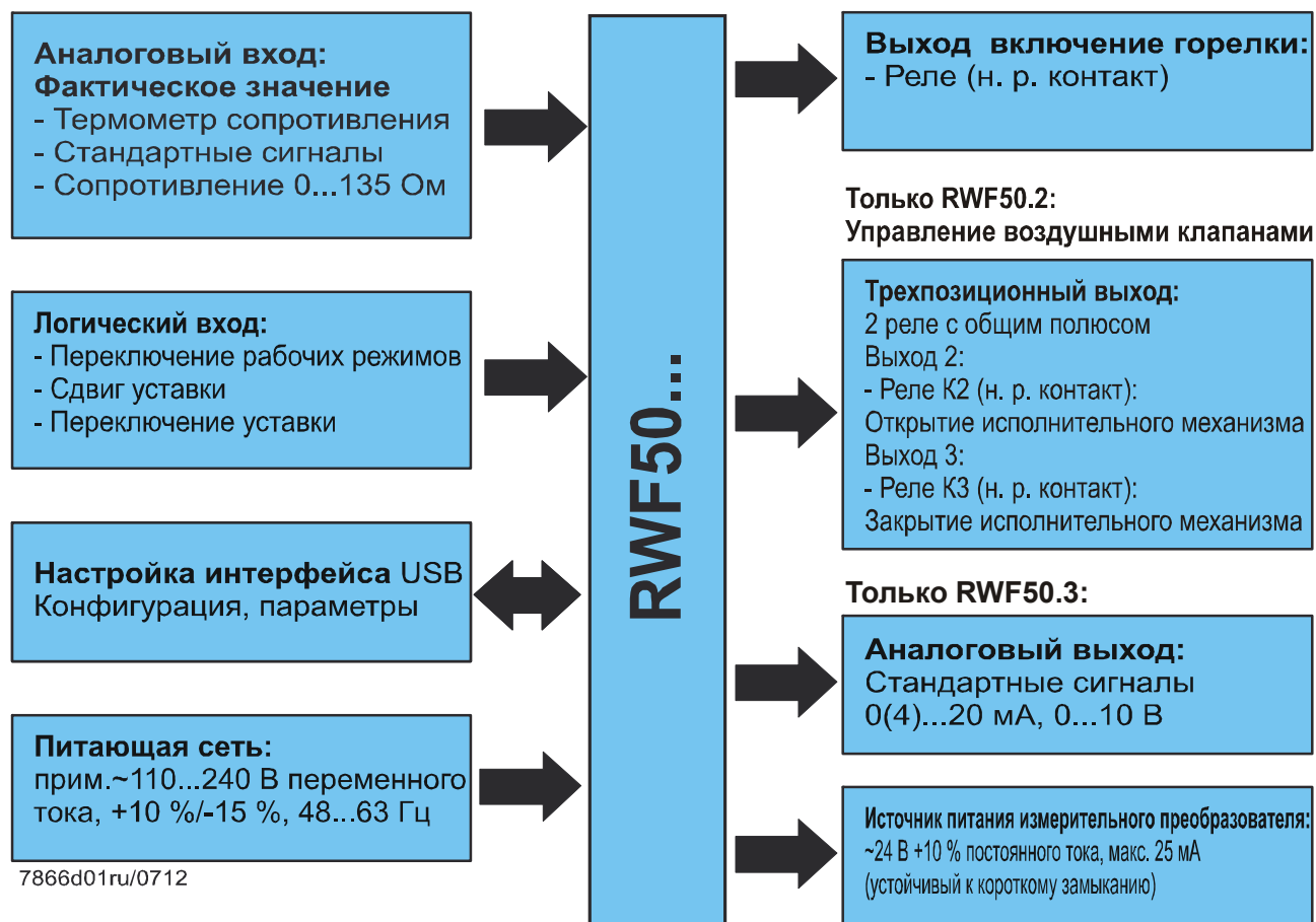
Иллюстрация 1: блок-схема
