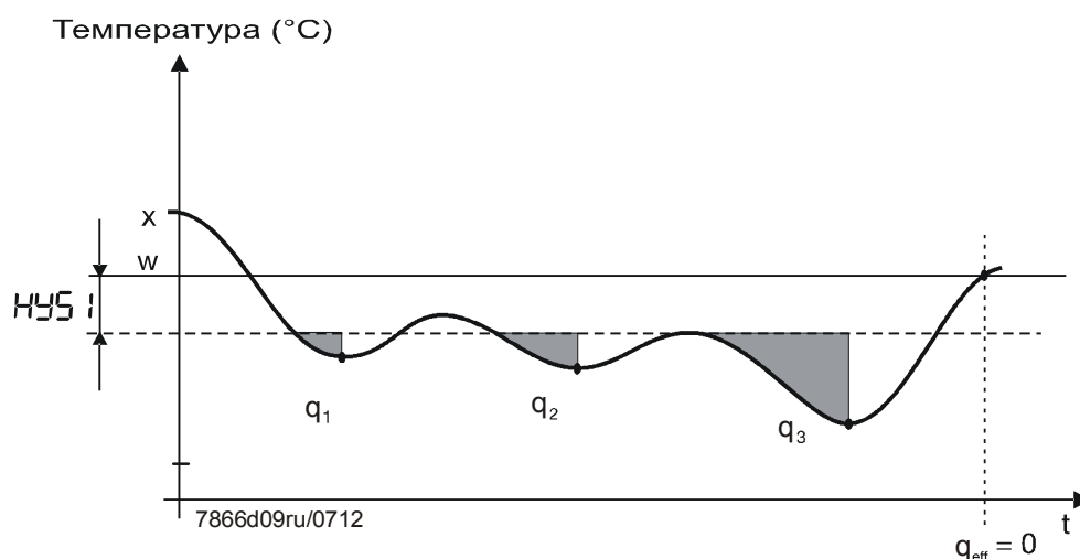
Иллюстрация 13: программируемый цикл горелки, порог срабатывания (q)
