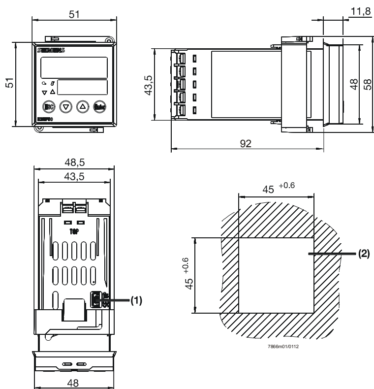
Иллюстрация 2: габаритные размеры RWF50
